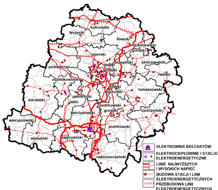
Rys. 53. System elektroenergetyczny w województwie łódzkim 2024 r.
