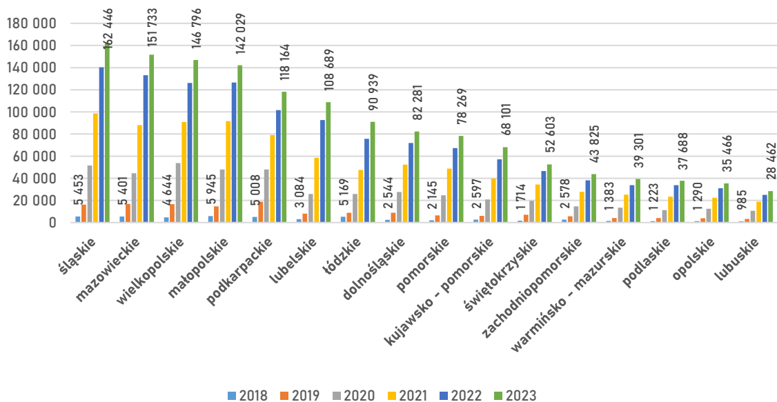
Wykres 31. Przyrost mocy zainstalowanej w mikroinstalacjach OZE w województwach w latach 2018–2023 [MW] (źródło: opracowanie własne na podstawie danych URE).
