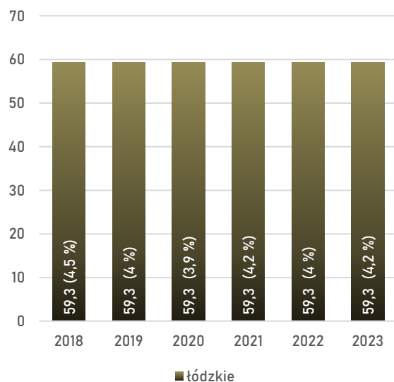
Wykres 26. Procentowy udział mocy elektrociepłowni i ciepłowni spalających biomasę w województwie łódzkim w mocy ze spalania biomasy w kraju w latach 2018 – 2023 [MW] (źródło: opracowanie własne na podstawie danych URE).
