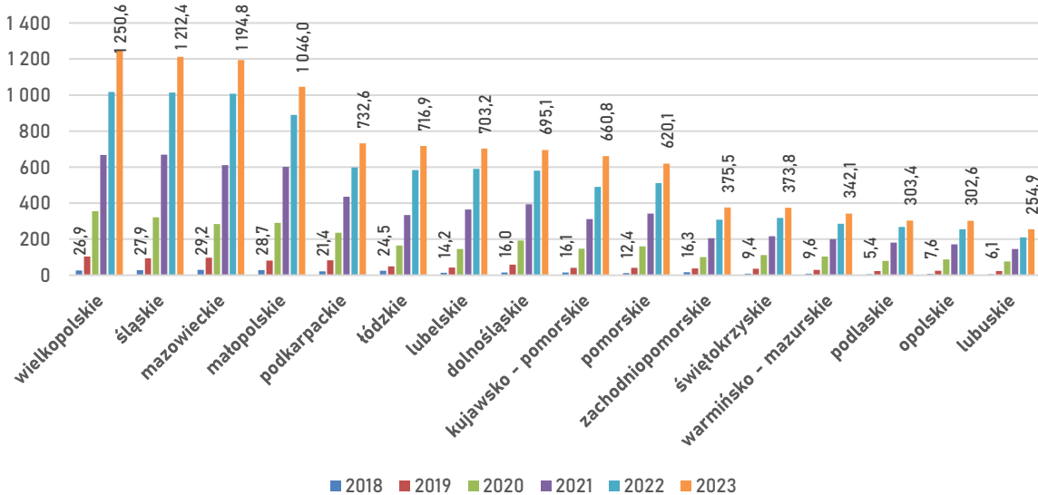
Wykres 31. Przyrost mocy zainstalowanej w mikroinstalacjach OZE w województwach w latach 2018–2023 [MW] (źródło: opracowanie własne na podstawie danych URE).
