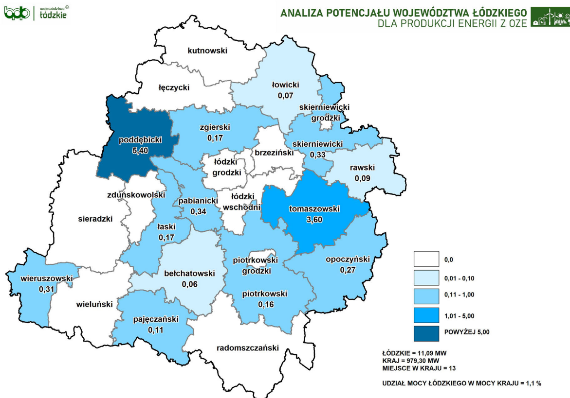
Rysunek 14. Moc instalacji wodnych w powiatach w 2018 r. [MW] (źródło: opracowanie własne na podstawie danych URE).
