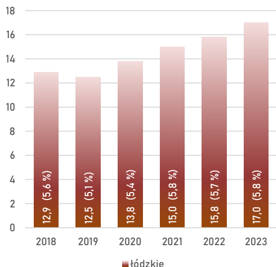
Wykres 22. Procentowy udział mocy instalacji biogazowych w województwie łódzkim w mocy instalacji biogazowych w kraju w latach 2018 – 2023 (źródło: opracowanie własne na podstawie danych URE).
