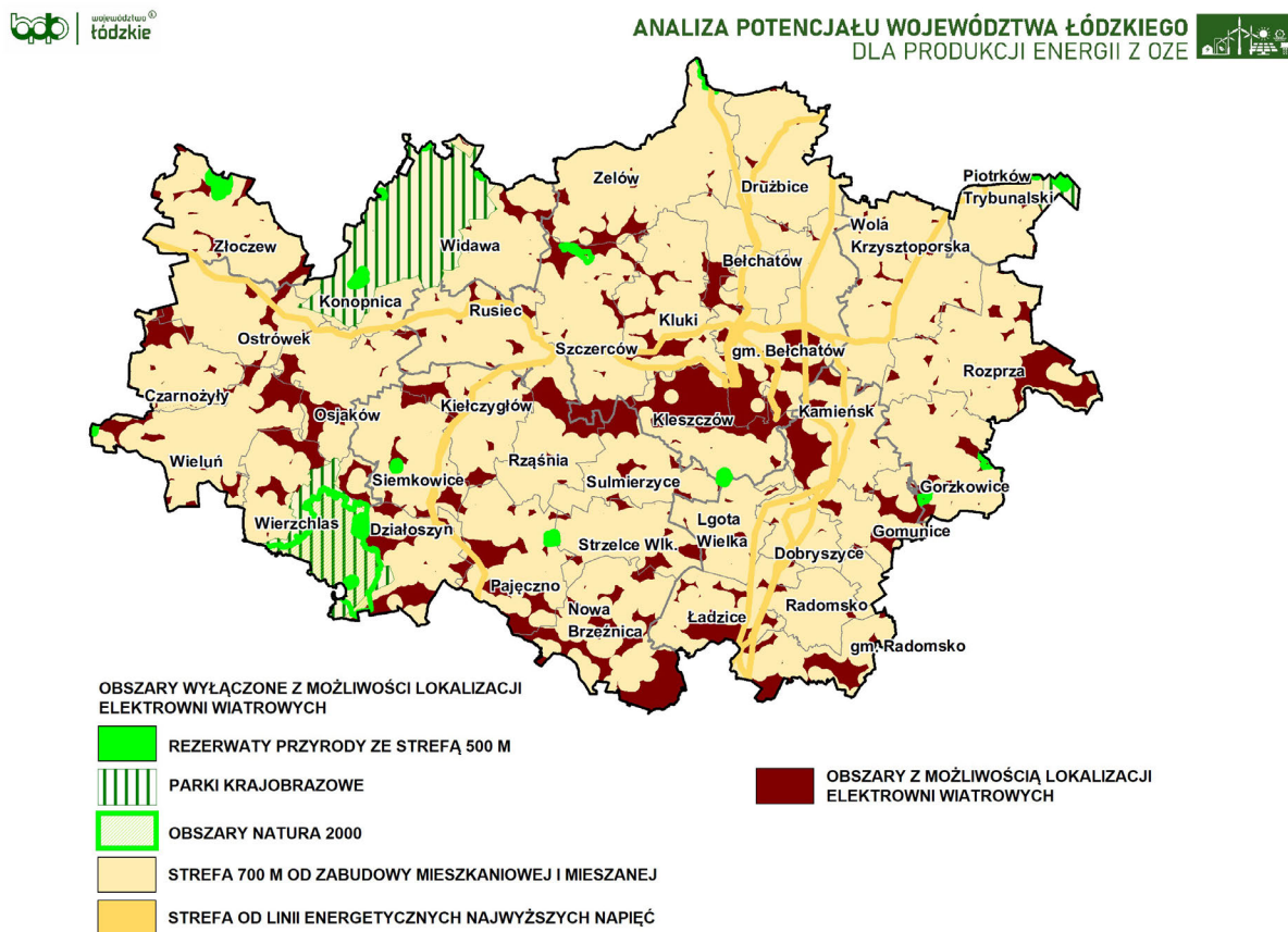
Rysunek 30. Możliwości lokalizacyjne nowych elektrowni wiatrowych na Obszarze Nowej Energii zgodnie z obowiązującą ustawą w 2023 r. (źródło: opracowanie własne na podstawie danych BPPWŁ).
